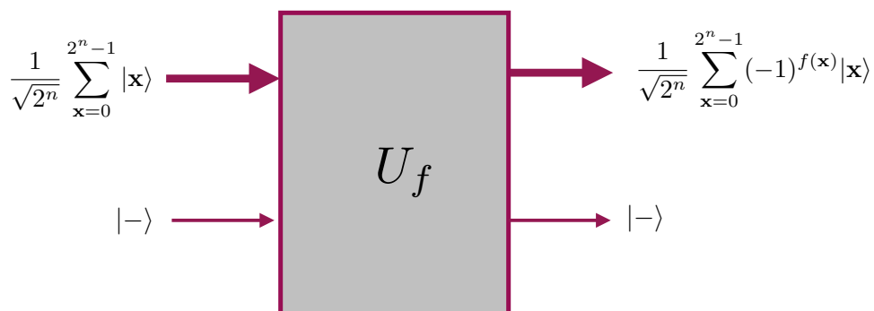
شکل ۲: مداری که برای الگوریتم دویچ - جوزا به کار می رود.
